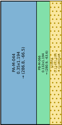
Pieza M-06 · 3 recorte(s)
