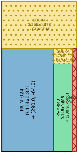
Pieza M-18 · 2 recorte(s)
