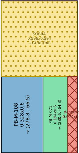
Pieza M-43 · 2 recorte(s)
